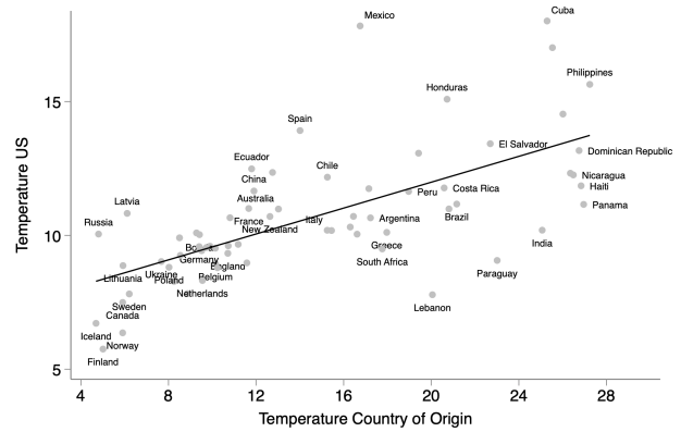
(d) 1940
